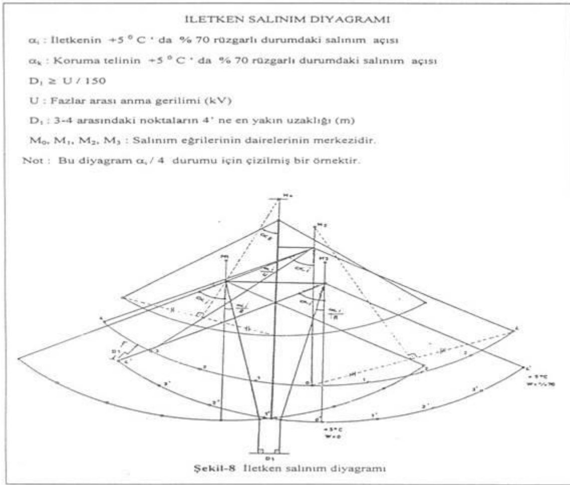
Şekil-8 İletken salınım diyagramı
