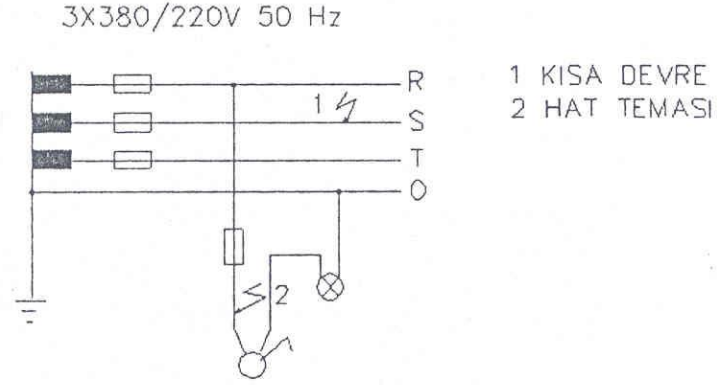
Şekil 3 - Kısa devre ve hat teması
