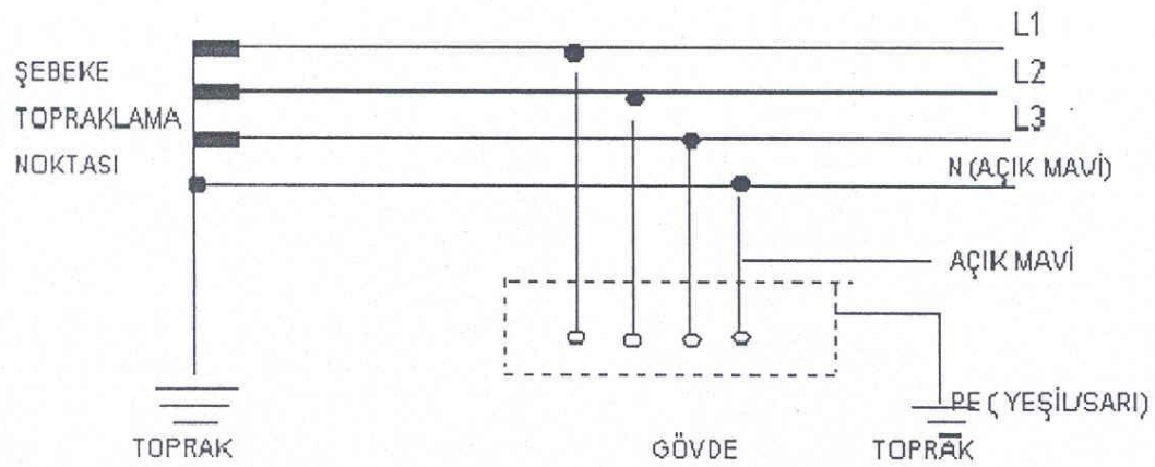
ŞEKİL 1-4 TT SİSTEMİ
